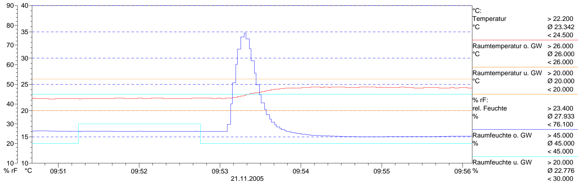
Raumklima Hygrotest 650 PHT
